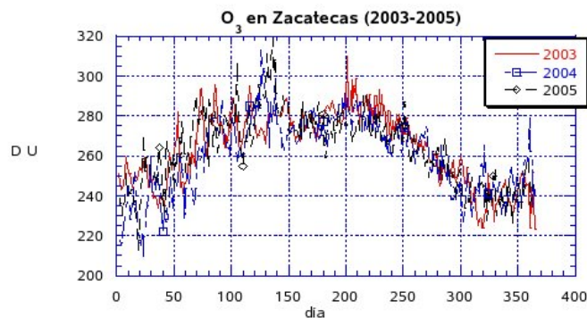
Figura 2. Comportamiento de la capa de ozono sobre Zacatecas entre 2003 y 2005, de acuerdo a TOMS [4].
